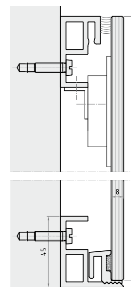
Magnetbefestigungssystem
