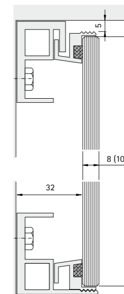
Standardbefestigungssystem
